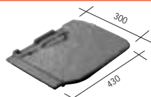
90 TL Right verge tile - 5 per m. - 2.75 kg.
