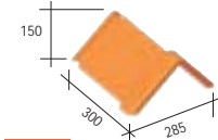
333 XT Flemish ridge tile - 4 per m. - 3.3 kg.
