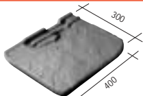
89 TL Left verge tile - 5 per m. - 3.75 kg.
