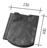
5 TL 1/2 tile - 2.4 kg.
