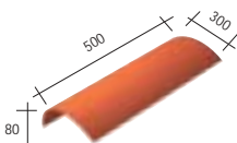
29 XG Ridge finish tile - 2.5 per m. - 5.3 kg.
