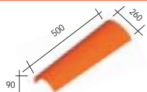
30 XG Non-interlocking ridge 500 mm - 2.5 per m. - 3.2 kg.
