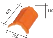
32 XG Angular ridge hip - 2.8 per m. - 3 kg.
