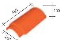
312 XG Circular ridge 400 mm - 2.5 per m. - 4.8 kg.
